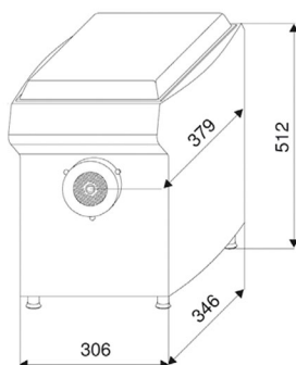
Dimensions Rubis
